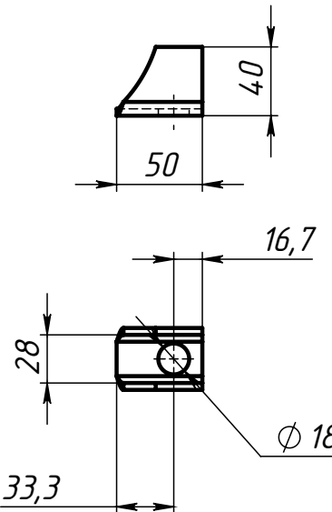
Поз.6 (Ушко)
