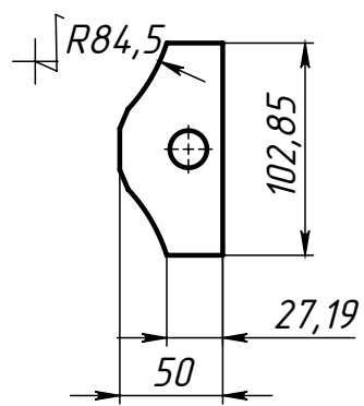
Поз.6 (Ушко) развертка
