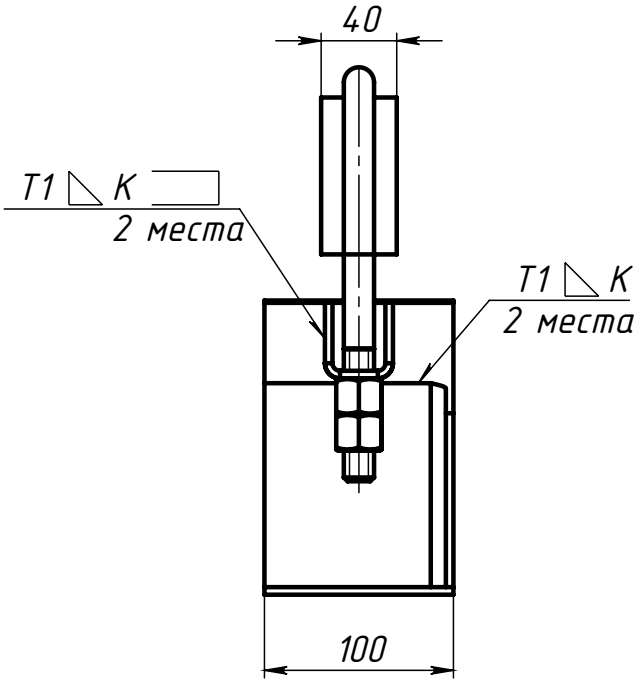
Поз.5 (Хомут)
