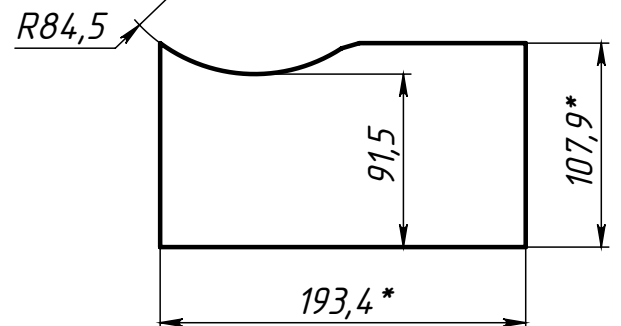
Поз.2 (Угольник) развертка
