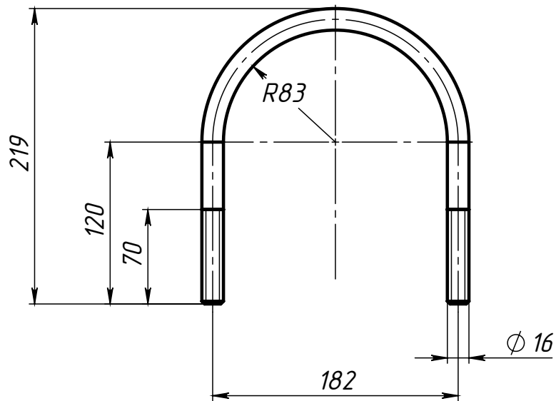
Поз.5 (Хомут)
