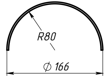
Поз.4 (Прокладка)
